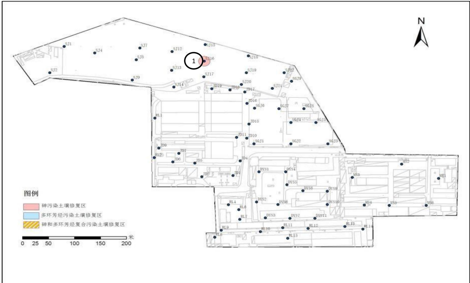
图 1.4-6 污染土壤第六层(5-6m)修复范围示意图
