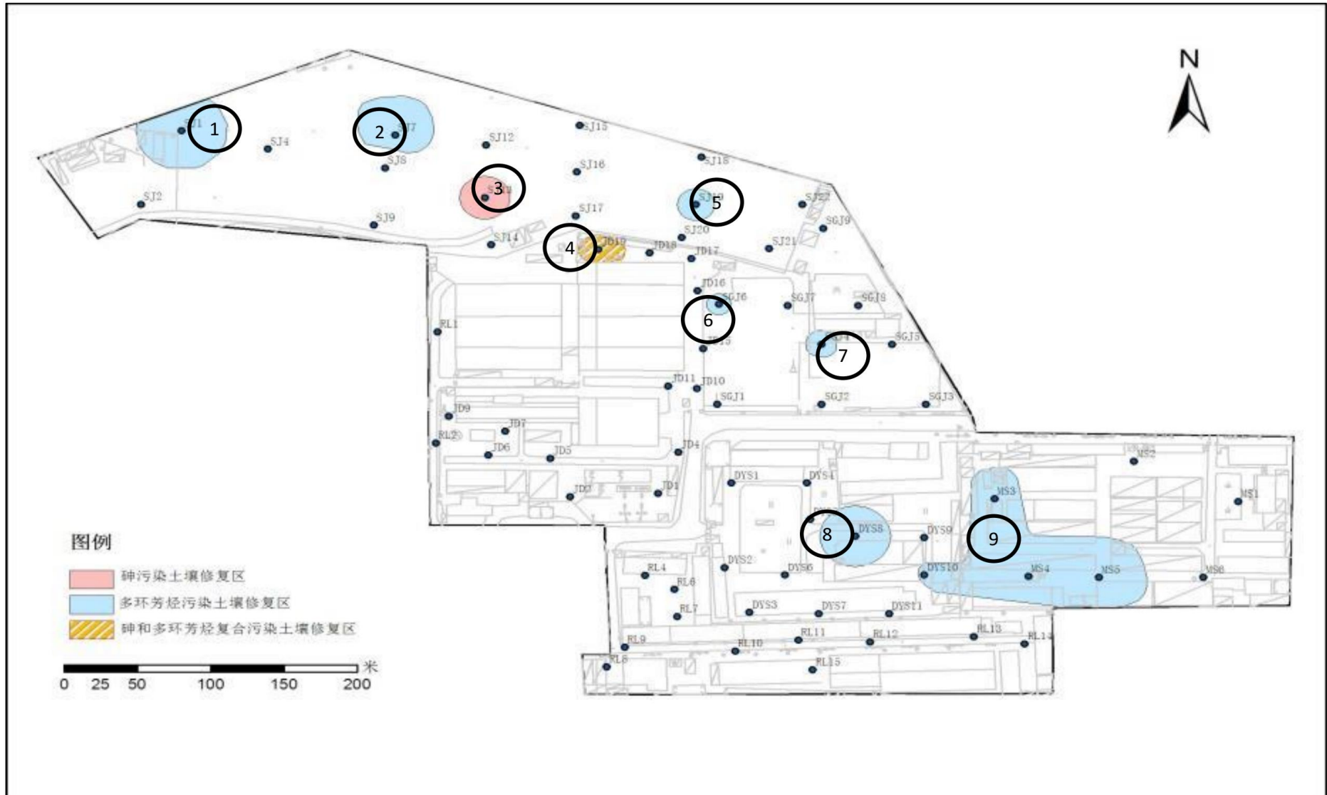
图 1.4-3 污染土壤第三层(2-3m)修复范围示意图
