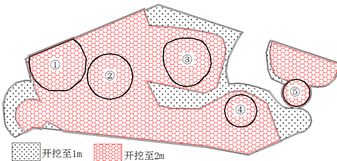
图 4.2-5 1#基坑第一层土开挖平面
