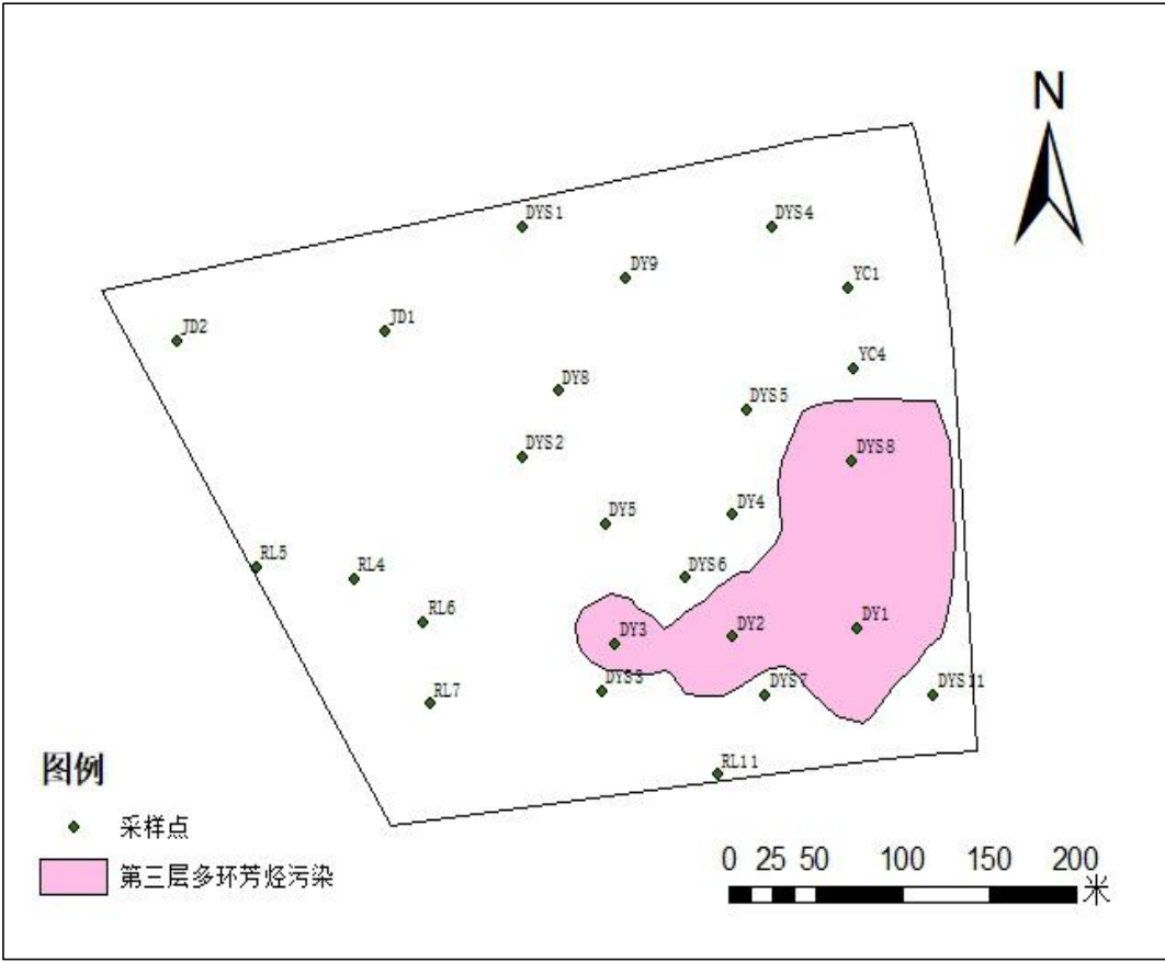
图 1.4-3 污染土壤第三层(2-3m)修复范围示意图
