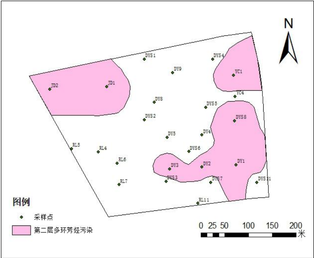
图 1.4-2 污染土壤第二层(1-2m)修复范围示意图
