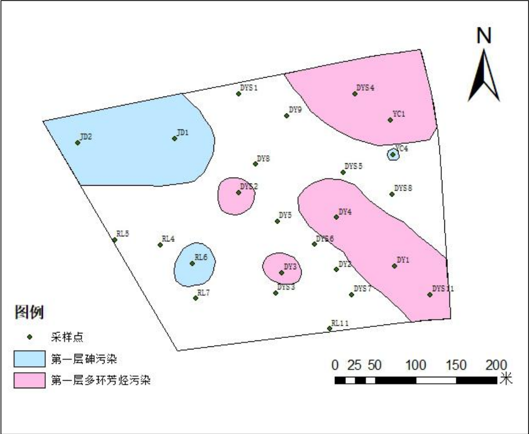
图 1.4-1 污染土壤第一层(0-1m)修复范围示意图
