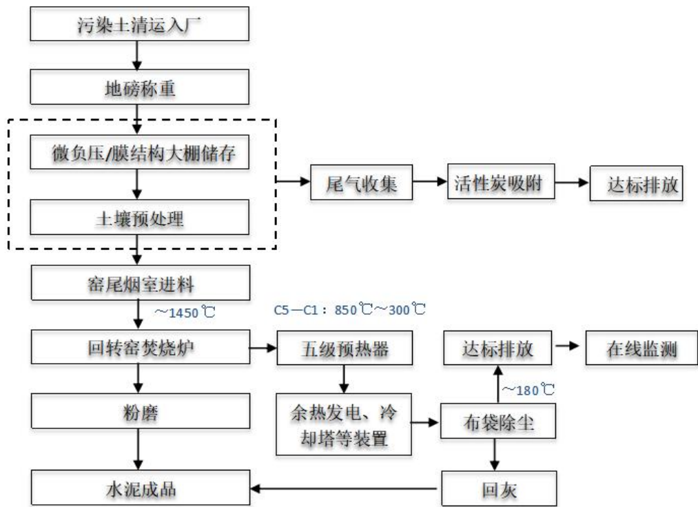
图 5.4-1 水泥窑焚烧处置技术工艺流程图
