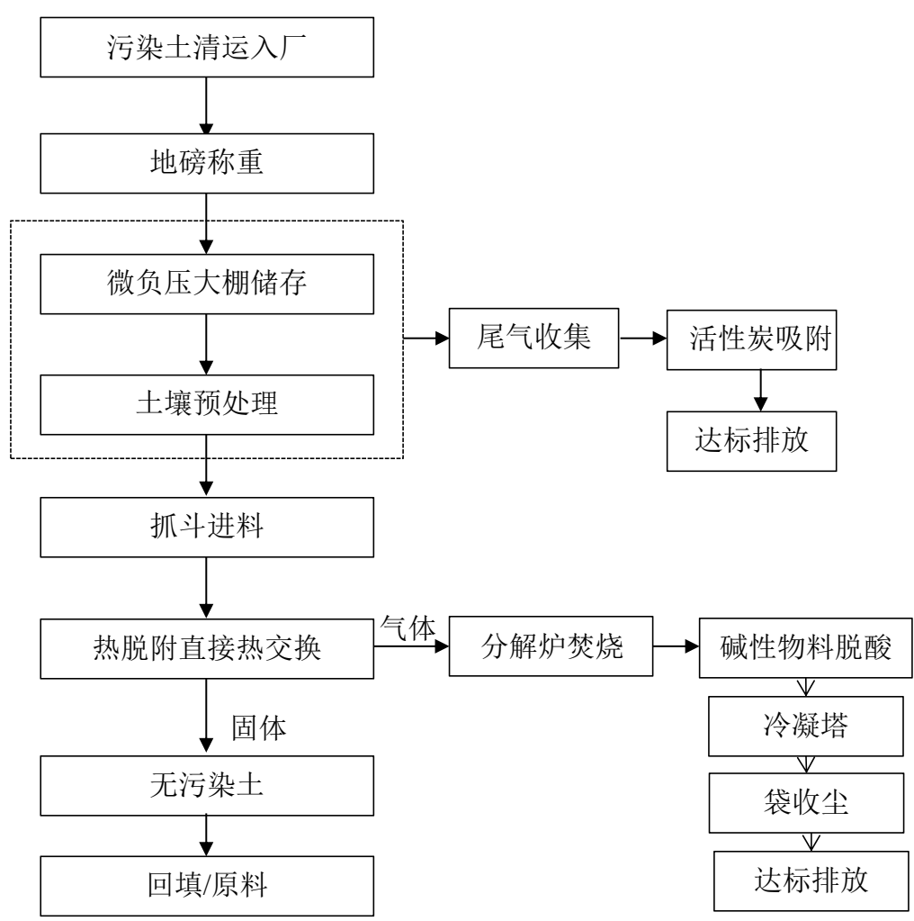
图 5.3-1 北京金隅北水环保科技有限公司污染土壤处置工艺流程图
