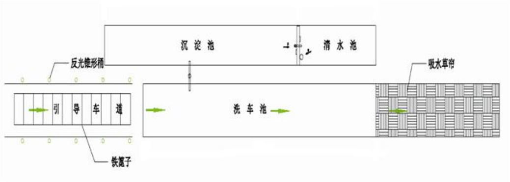
图 3.1-1 环保洗车循环系统平面图
