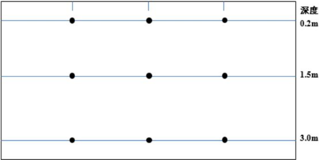
图 7.4-3 基坑侧壁系统布点法
