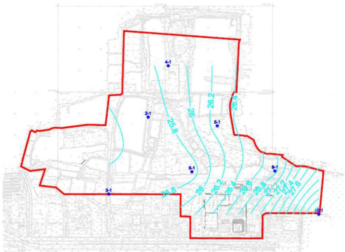
图 5.3-3 第一层地下水标高等值线图
