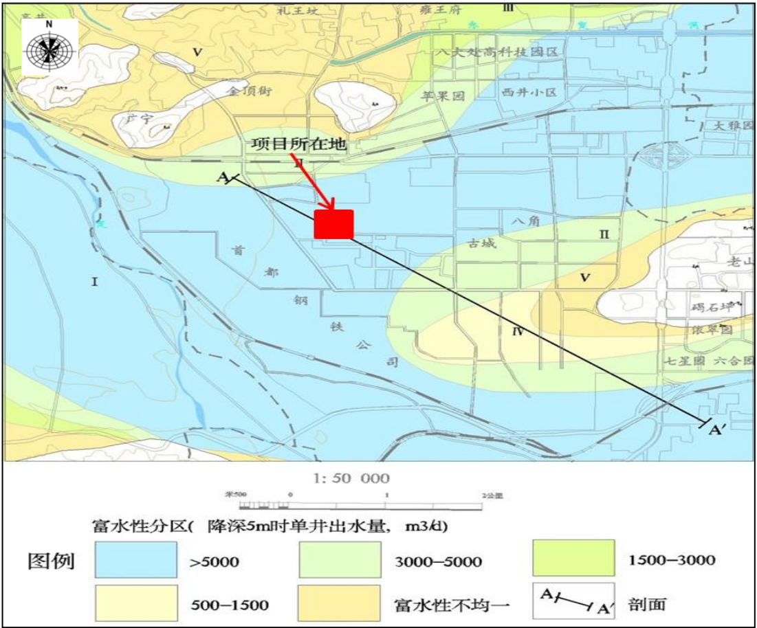
图 3.2-3 区域第四系水文地质图
