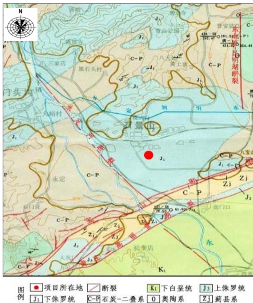
图 3.2-1 项目所在区域基岩构造图
