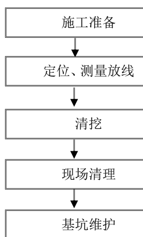
图 5.2-3 污染土壤清挖工艺
