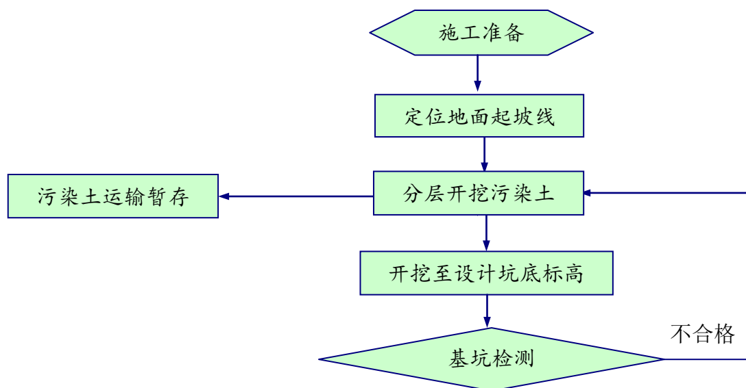
图 4.2-10 土壤清挖流程
