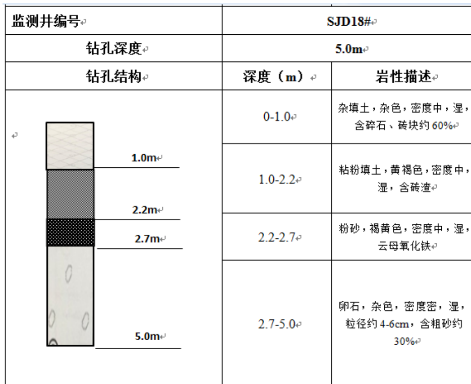
图 1.4-1 钻孔柱状图
