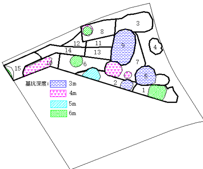
基坑分区与3m深以上基坑对比图
