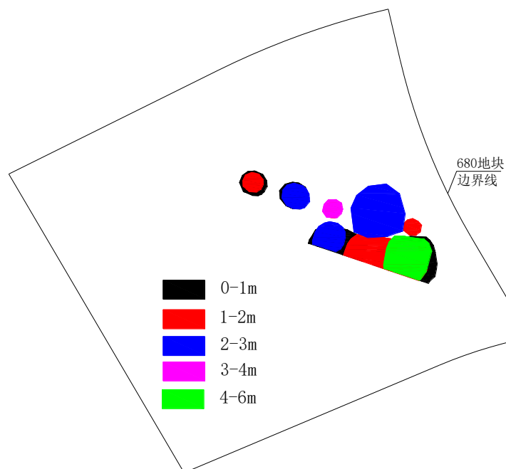
图 4.2-3 680-1 地块砷污染土、多环芳烃及砷复合污染土分层清挖图
