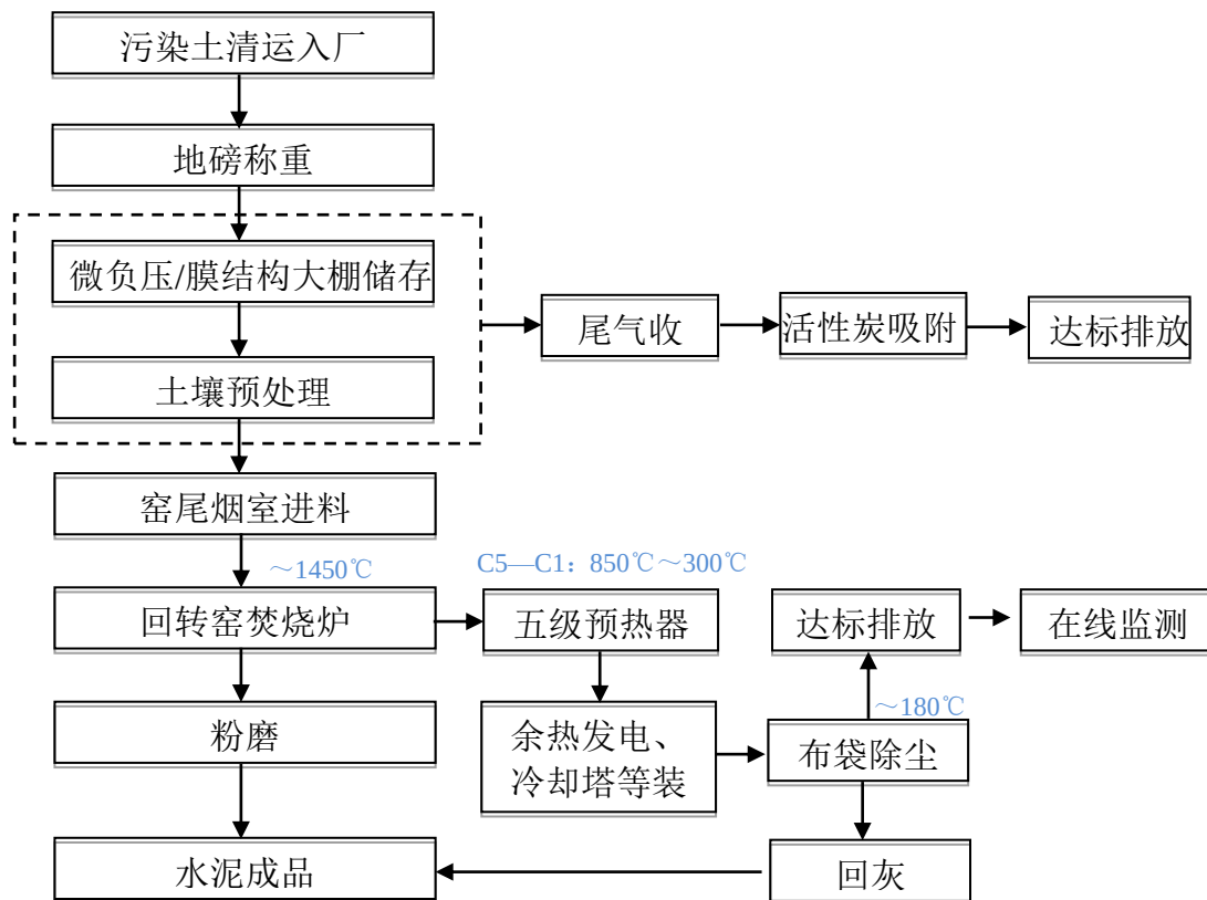
图 5.4-1 水泥窑共处置技术工艺流程图
