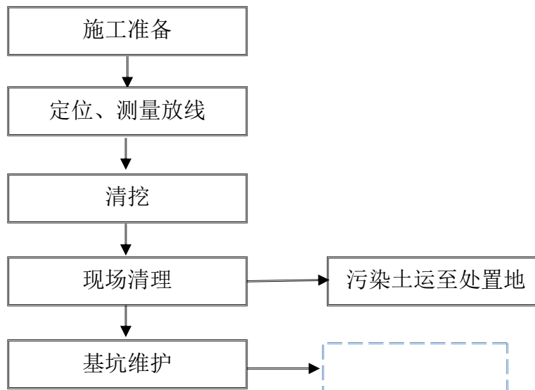
图 4.2-1 污染土壤现场清理及运输工艺流程
