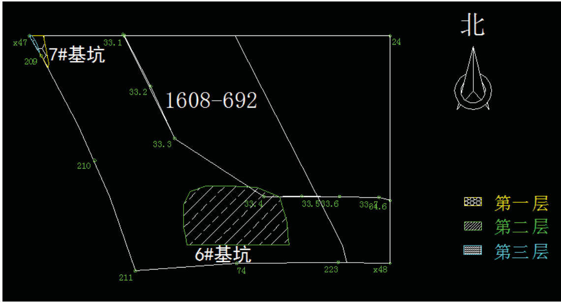
图 15.2-1 692 地块污染土分层图
