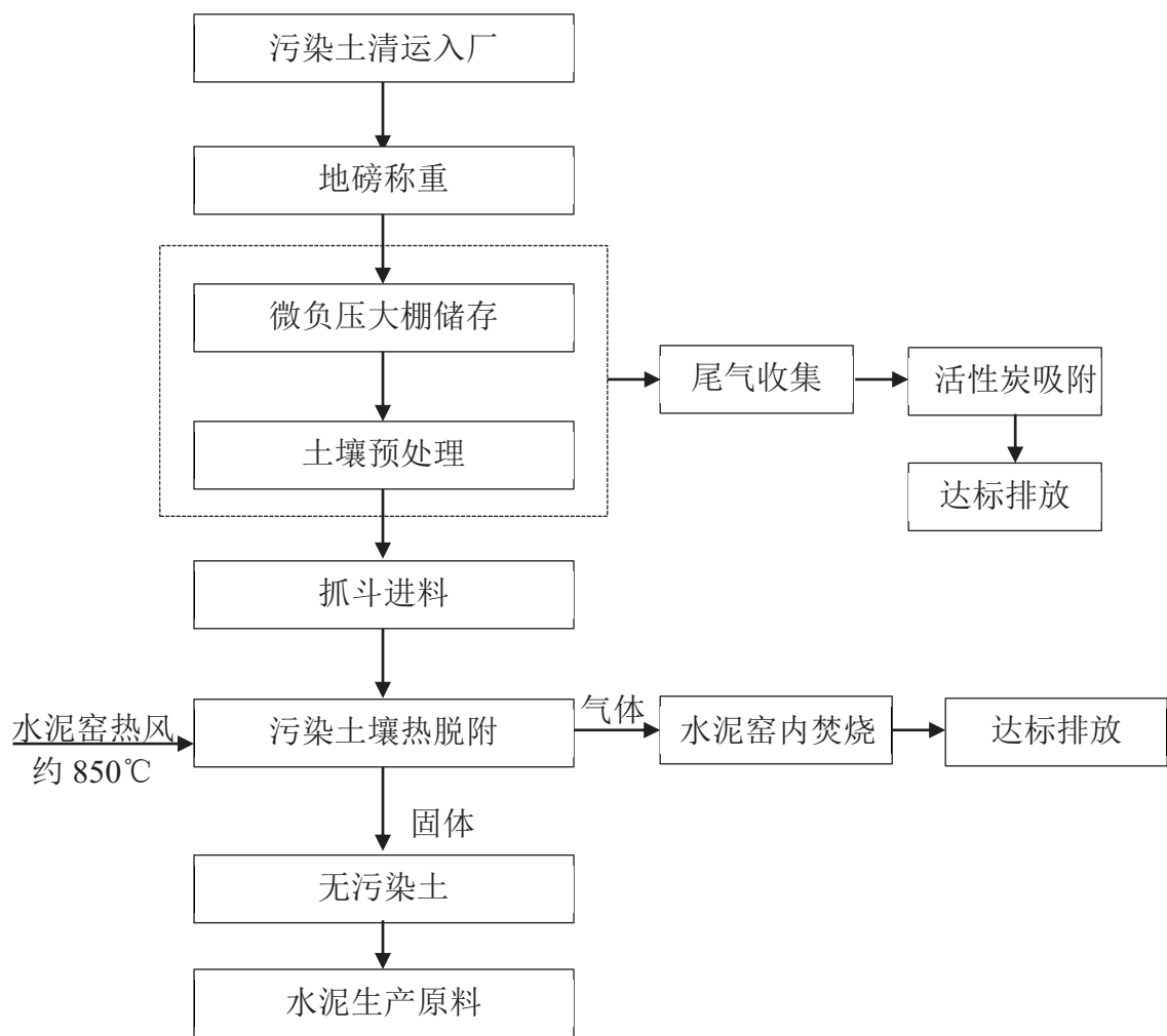
图 5.3-1 北京金隅北水环保科技有限公司污染土壤处置工艺流程图
