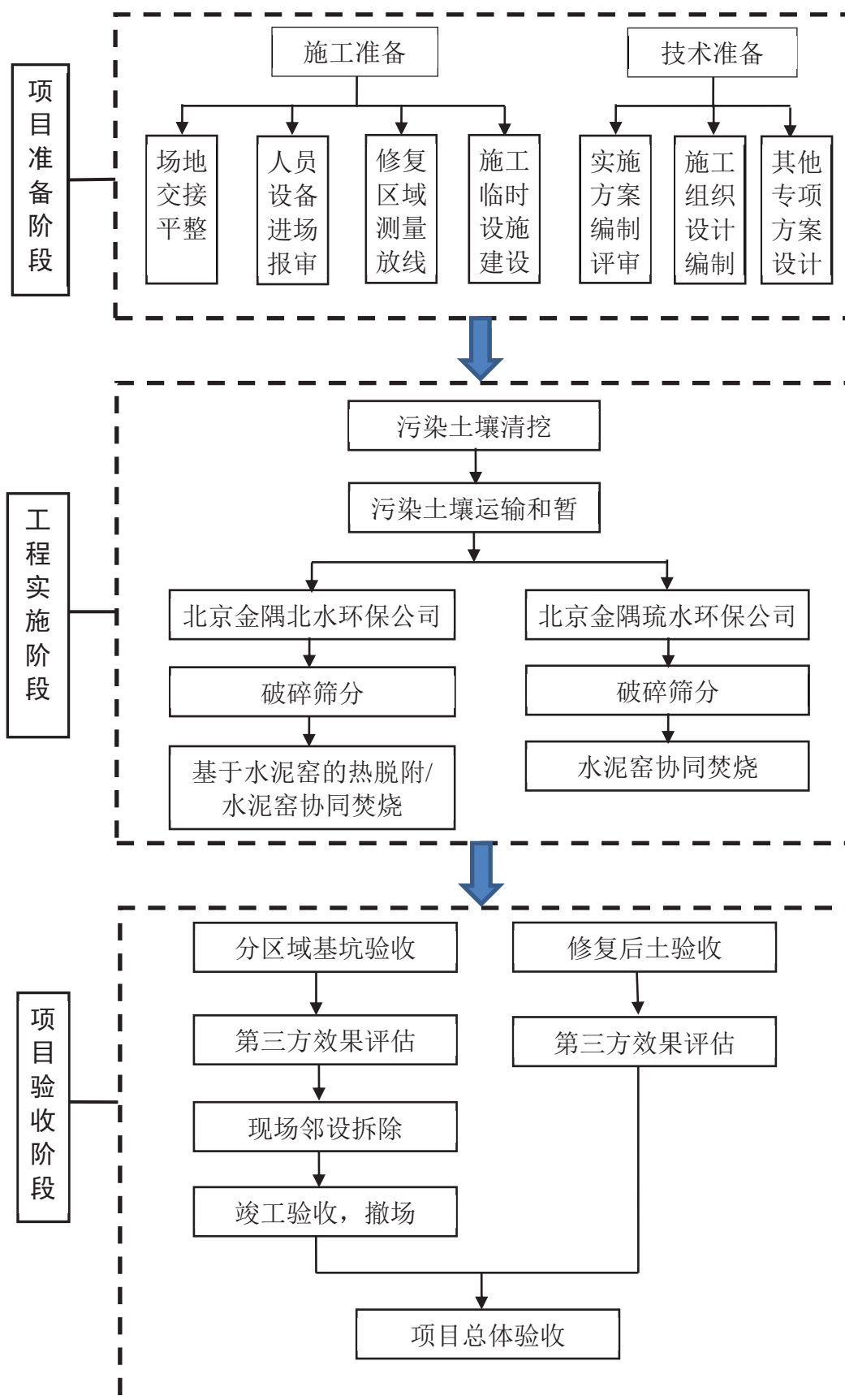
图 3.2-1 主要施工流程图
