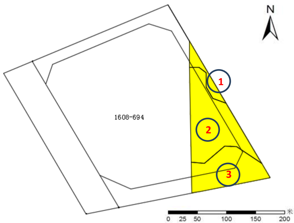
图 8.2-1 污染土第一层（0-1m）修复示意图
