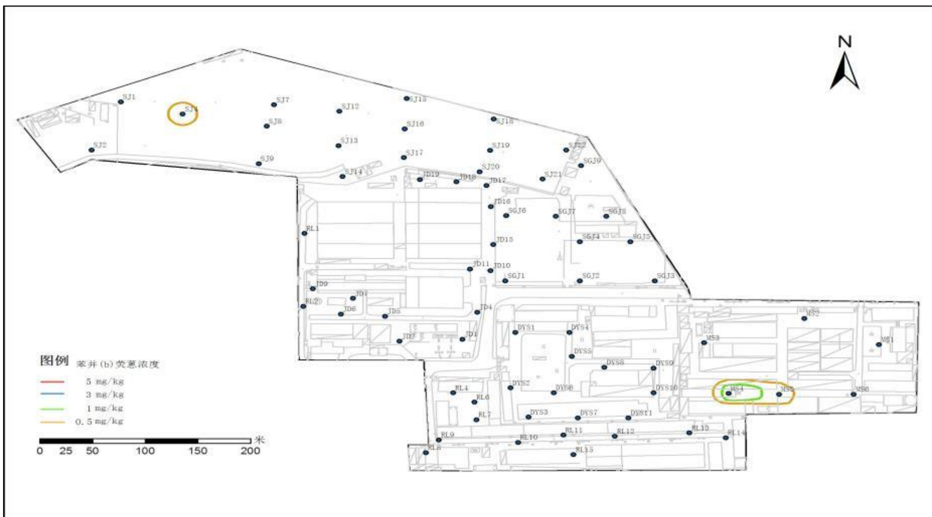
图 4.2-29 埋深 4-5m 范围内土壤样品中苯并(b)荧蒹浓度分布示意图
