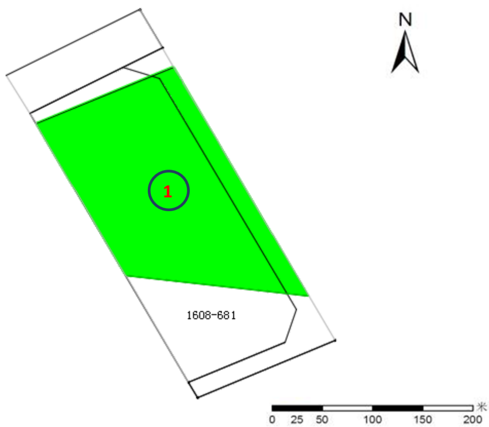
图 8.2-2 污染土第二层（1-2m）修复示意图
