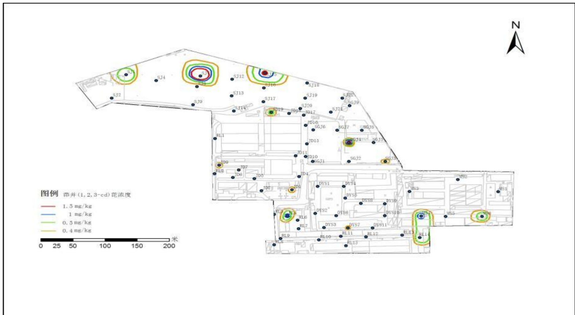
图 4.2-38 埋深 1-2m 范围内土壤样品中卽并(1,2,3-cd)茈浓度分布示意图
