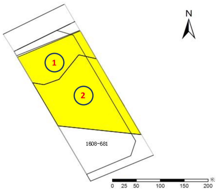
图 8.2-1 污染土第一层（0-1m）修复示意图
